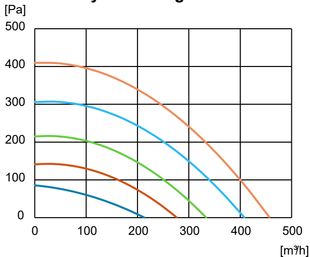
Nyomás / Légszállítás
