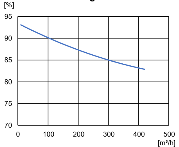
Hatásfok / Légszállítás
