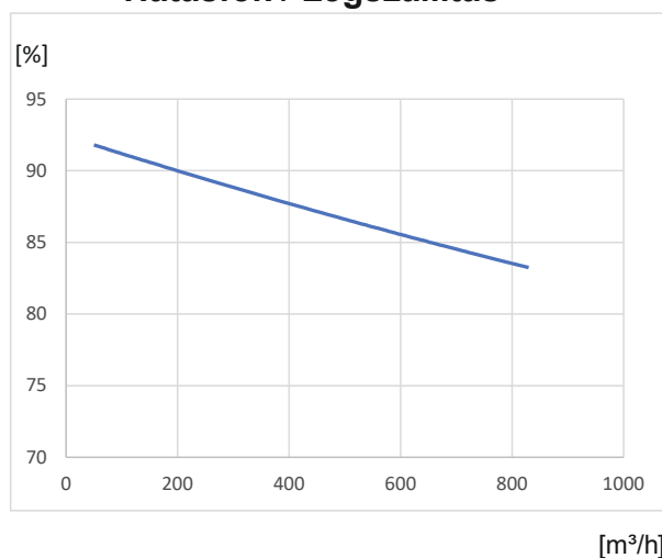
Hatásfok / Légszállítás
