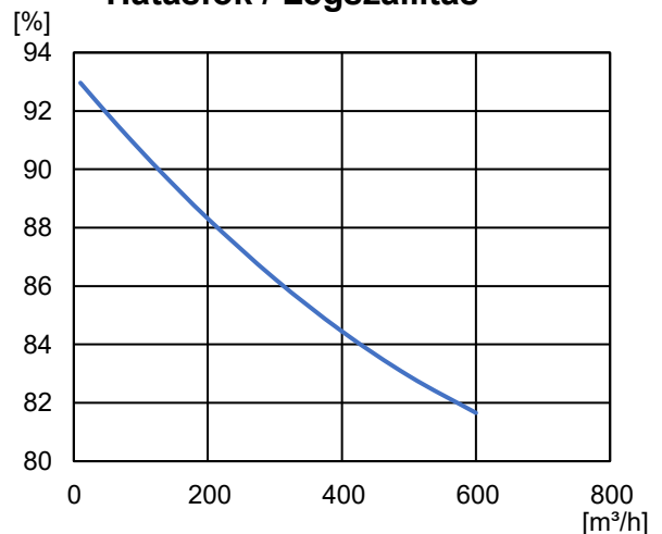
Hatásfok / Légszállítás
