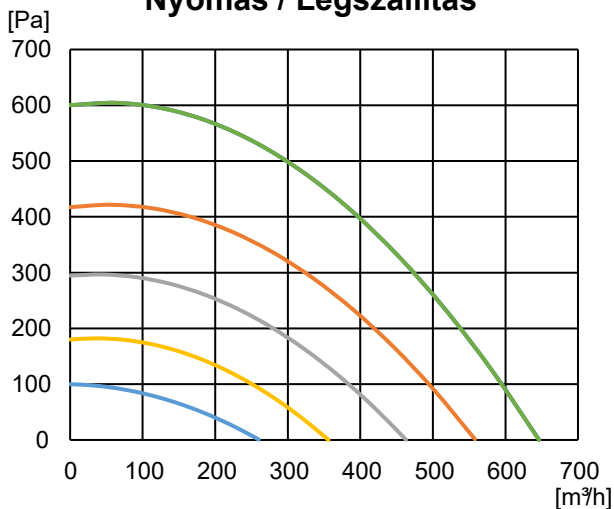
Nyomás / Légszállítás
